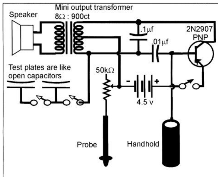
Syncrometer® Schematic
